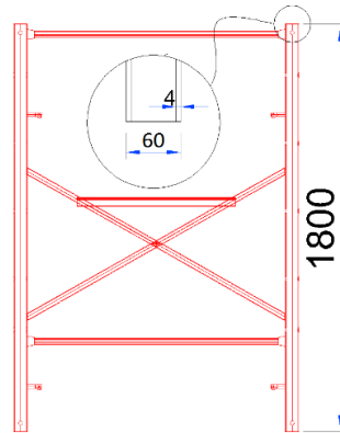
Shorbrace Frame
